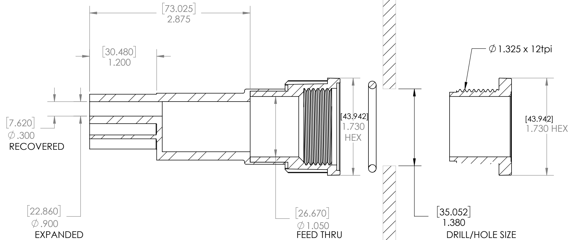
SECTION A-A SCALE 1 : 1
